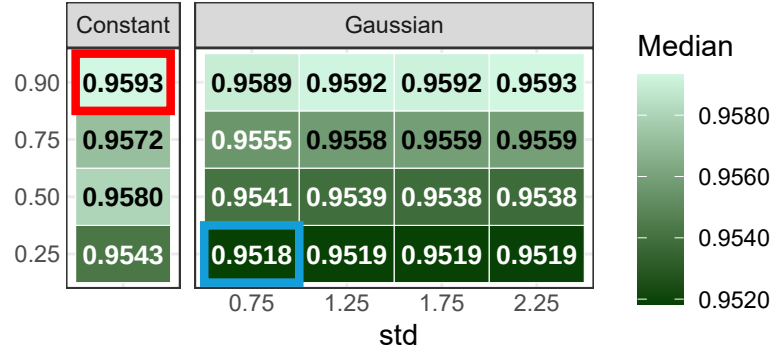
FDR
