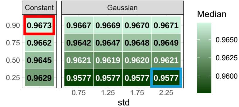
NPV
