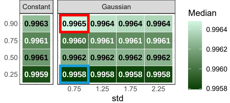
Precision
